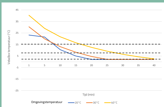
Terugkoelprestatie bij verschillende omgevingstemperaturen Model C Cool
