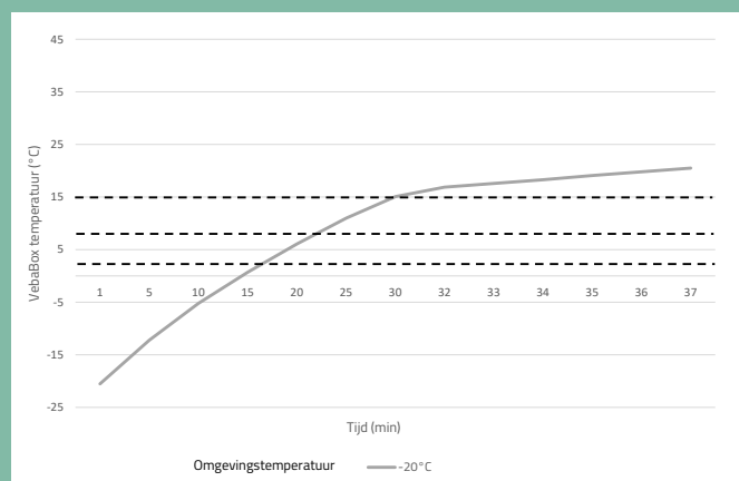
Verwarmingsprestatie bij omgevingstemperatuur Model C Cool
